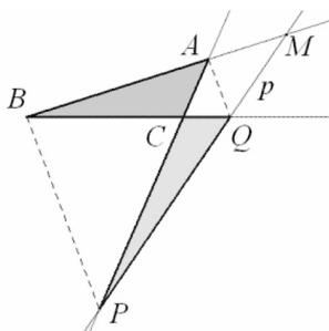
Poslední vztah umožňuje sestrojit úsečku délky d = |CP| jako čtvrtou geometrickou úměrnou podle obr. 3. Bod P pak v zadání úlohy narýsujeme nanesením délky d na polopřímku opačnou k polopřímce CA . Bod Q je průsečík přímek MP a BC .
