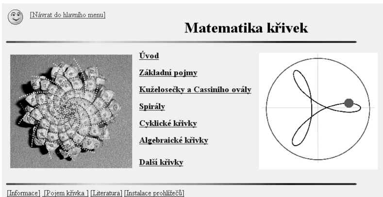
Obr. 2: Matematika křivek
